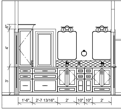
E1 ENSUITE CABINETS 3/16 in = 1 ft
